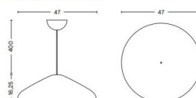
Pao Steel Pendant 470
