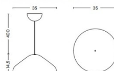
Pao Steel Pendant 350
