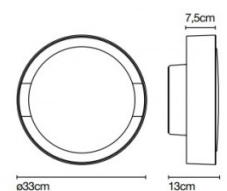
Plaff-on! 33 IP54
